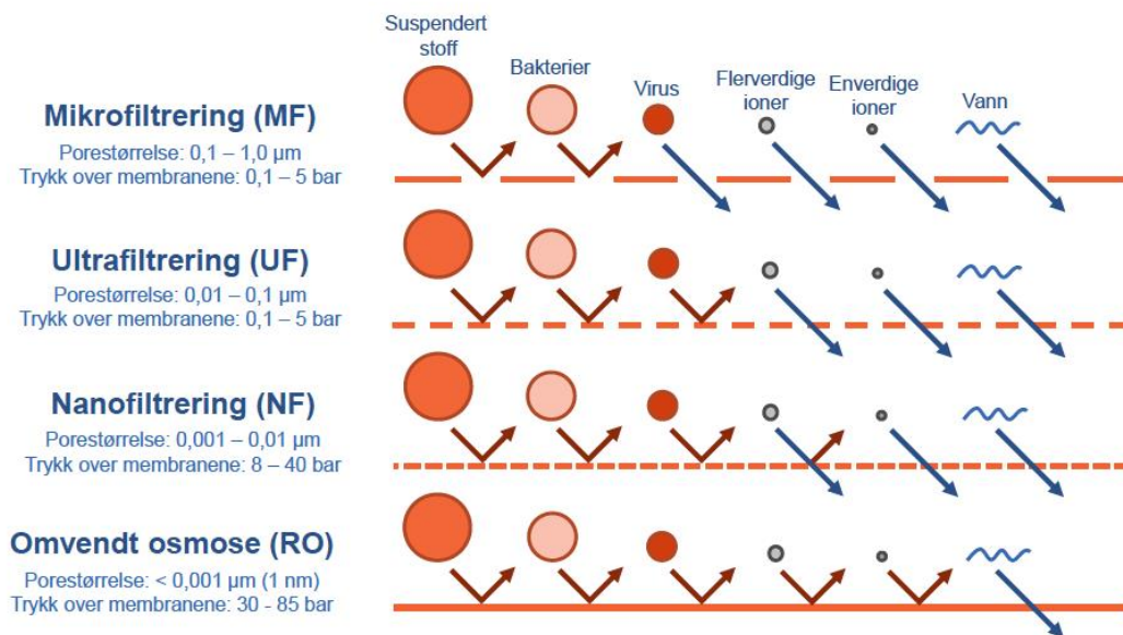
Figur 1. Forskjellige filtreringsprosesser
